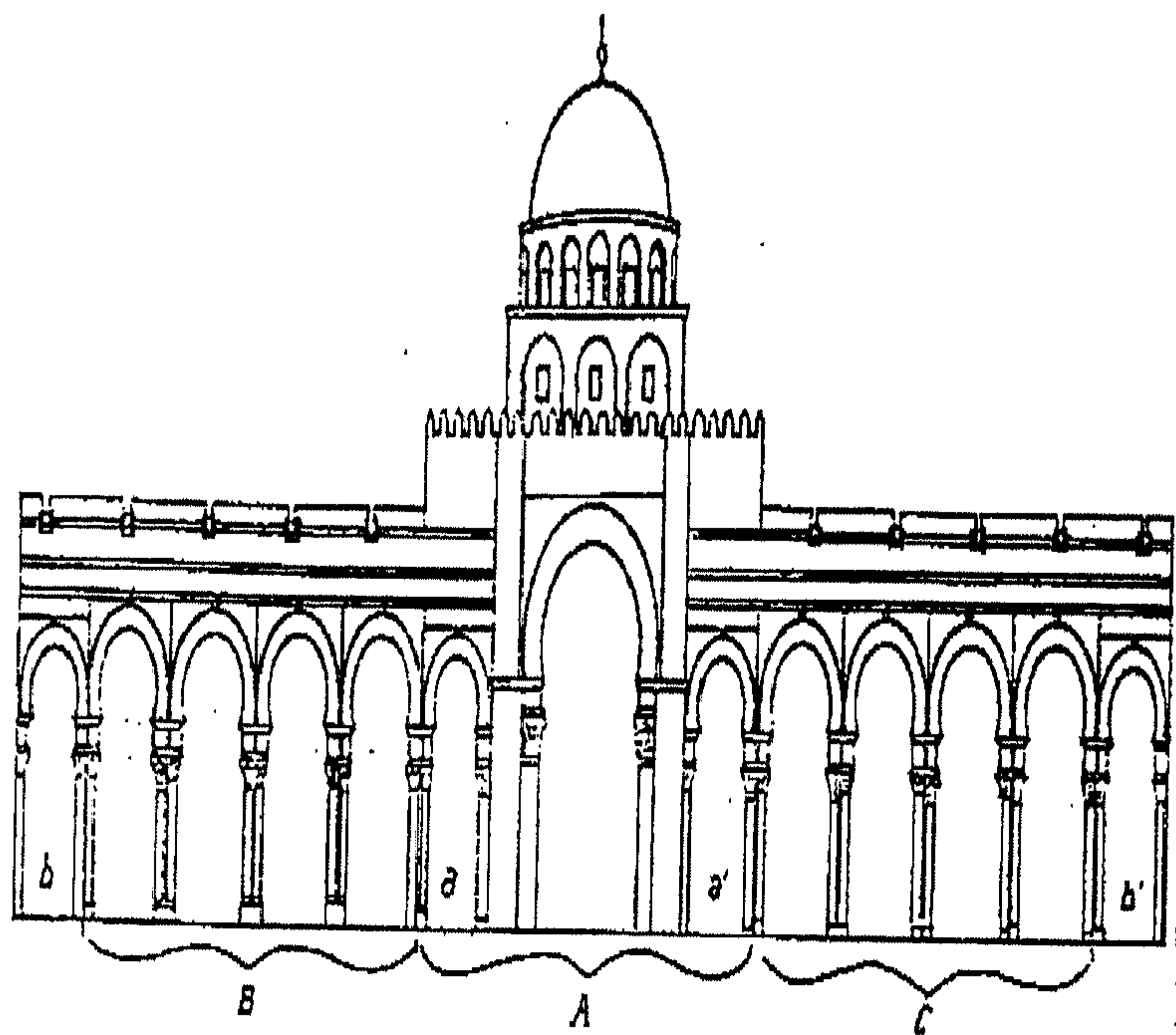
(شكل رقم ١٤) واجهة مقدم جامع القيروان في عهد ابراهيم الثاني بن أحمد عن ليزين
